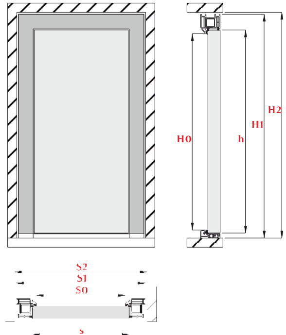
Durų schema be užlaidos
