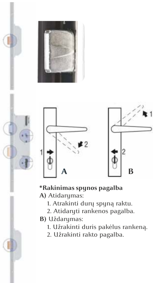
Trijų taškų juostinė spyna SECURITY EUROPA MR2
