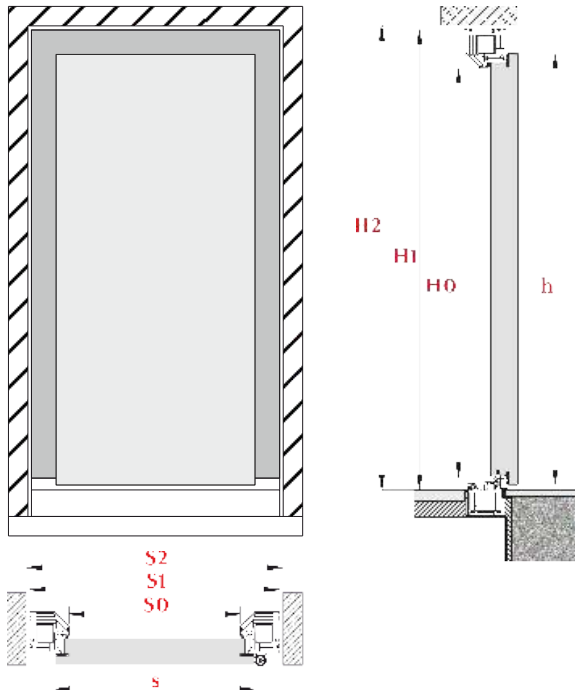
Durų schema su užlaida
